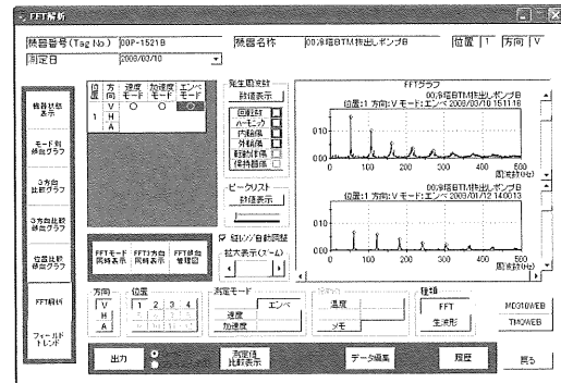
図 13. 発生周波数確認画面
