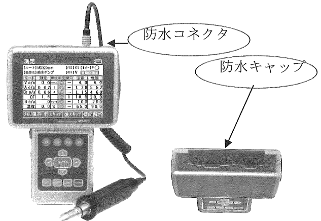
図 8. 防塵・防滴構造
