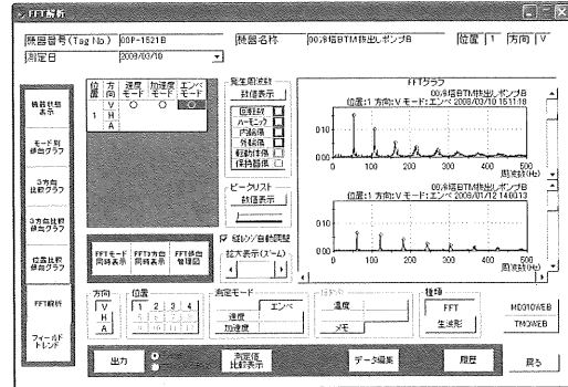
図 12. FFTデータ比較画面
