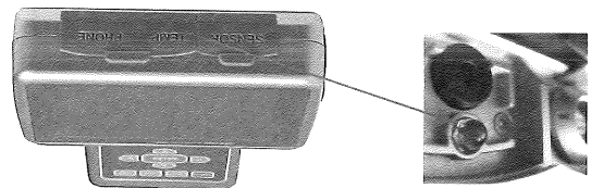
図 9. 非接触式赤外線温度センサ
