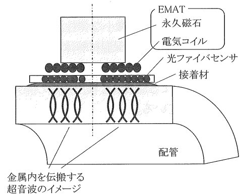
図10 センサ構造
