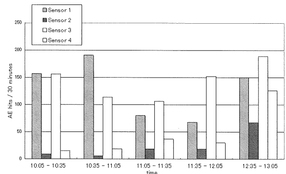
図7 実機反応器
