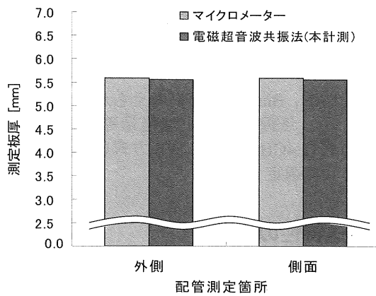
図 13 100A エルボ配管の肉厚測定結果
