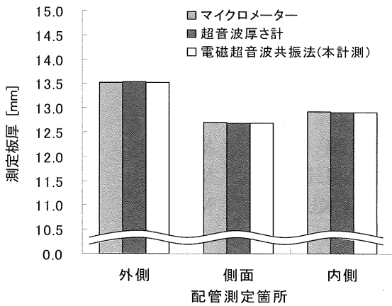
図 12 250A エルボ配管の肉厚測定結果
