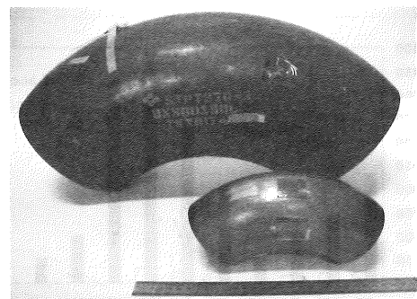
図11 試験に用いた配管エルボサンプル (奥側:250A、手前側:100A)
